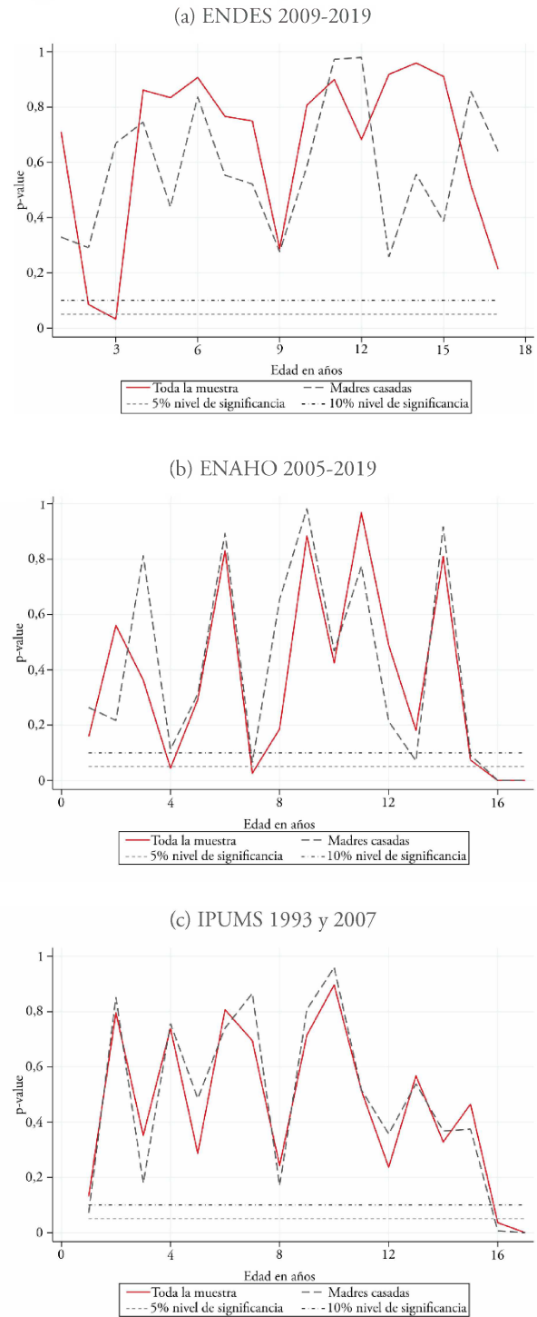
Figura C1. Prueba conjunta del estadístico F
