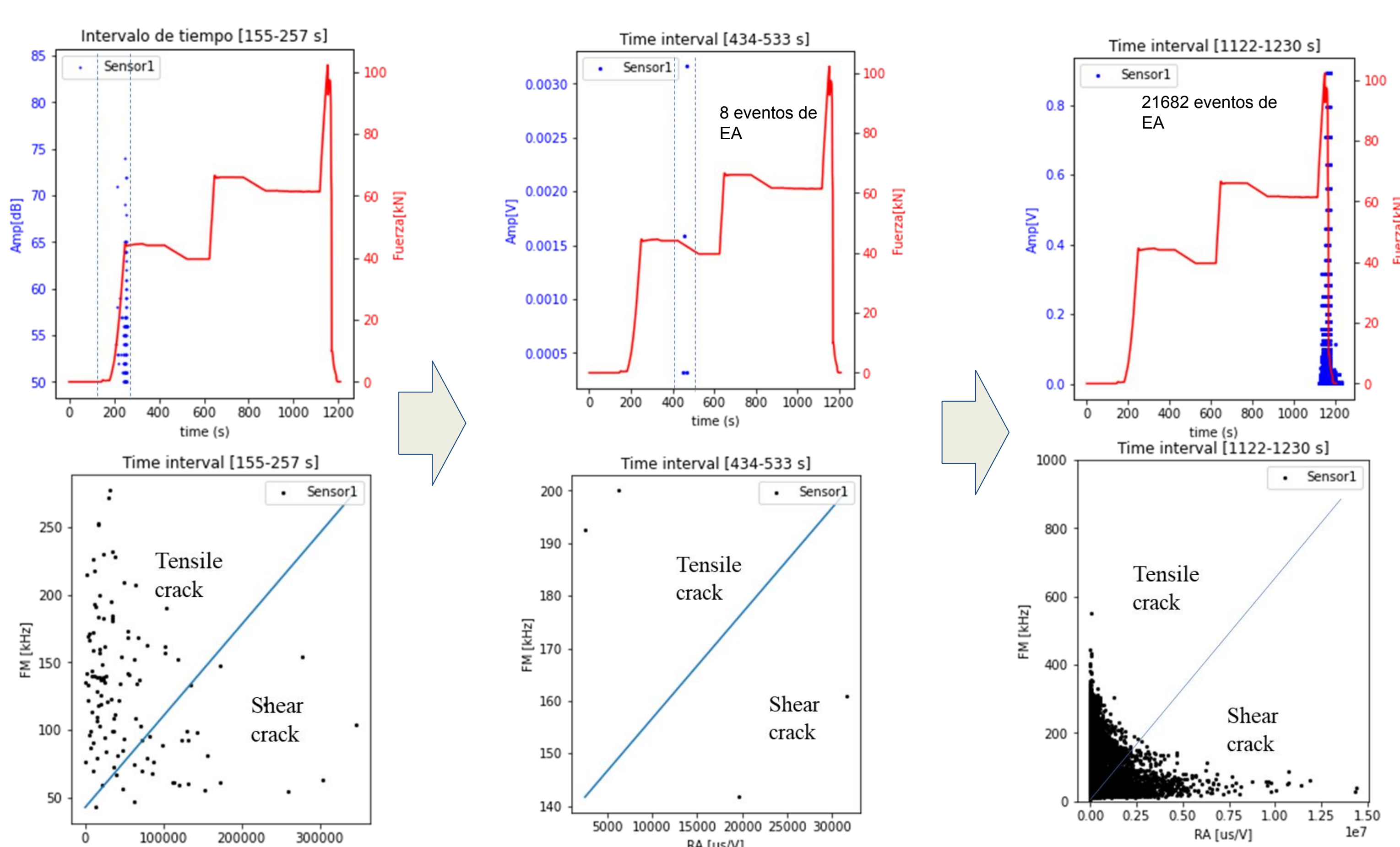
Fig 5. Para analizar los modos de ruptura predominantes (Tensil o Corte) durante las diferentes etapas del ensayo se calcularon las tendencias de los parámetros secundarios RA= RiseTime/Amplitud y la frecuencia media FM=Cuentas/Duración, ver ref [4].
