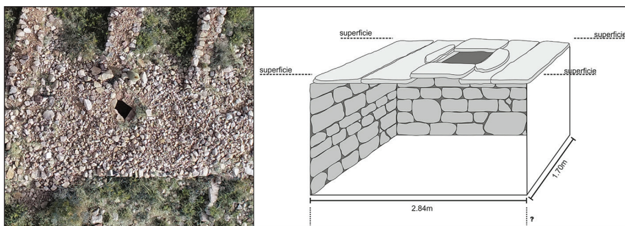
Figura 8. Izquierda: fotografía aérea de un despietre donde se observa la apertura de un granero; derecha: representación esquemática del granero
