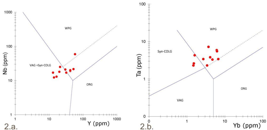
Figura 2: a) Diagrama Y-Nb, b) Diagrama Yb-Ta. El Granito Peñas Blancas se vincula en parte a un ambiente de intraplaca (WPG) y en parte a un ambiente colisional (COLG). Pearce et al. , (1984).
