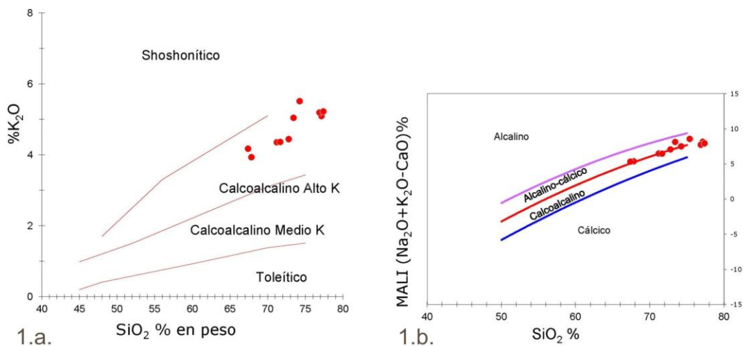
Figura 1: a) Diagrama SiO 2 vs. K 2 O según Le Maitre (1989). b) Índice de alcalinidad modificado SiO 2 vs. (MALI) según Frost et al. (2001).
