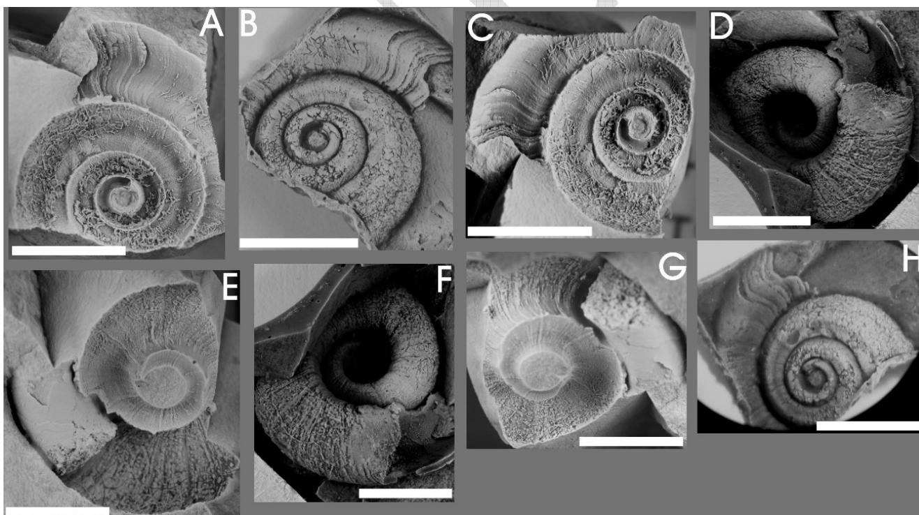
Figura 6. Euomphalus tenuicarيناتus sp. nov. A-H. A. MLP 26167, Holotipo, molde externo, vista apical, detalle de lamelas de crecimiento; B. MLP 26167, Holotipo, molde de látex, vista apical oblicua, detalle de la protoconcha con gap central; C. MLP 26167, Holotipo, molde de látex, vista apical, detalle de la protoconcha con gap central; D. MLP 26166, molde de látex, vista basal; E. MLP 26166, molde externo, vista basal; F. MLP 26166, molde externo vista basal; G. MLP, molde externo, vista basal; H. MLP 26167, Holotipo, molde de látex, vista apical. Escala grafica=10mm.
