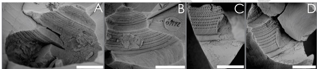
Figura 4. Glabrocingulum (Stenozone) heminodosus nov sp. A-D. A. Holotipo MLP 26143, molde externo; B. MLP 26149, molde externo, detalle de la ornamentación espiral en el perfil superior de la vuelta, selenizona, perfil exterior con líneas de crecimiento en la última vuelta; C. MLP 26148, molde externo última vuelta, detalle de la ornamentación espiral con nodos en el perfil superior y solo líneas de crecimiento en el perfil exterior, selenizona y lúnulas; D. MLP 26148, molde externo, detalle de la ornamentación en la última vuelta. Escala gráfica= 10mm.
