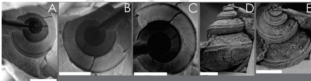
Figura 5. Lagunaspira labrocostellata gen et sp. nov. A-E. A-C, MLP 26168, concreción, molde externo, detalle de las vueltas, ornamentación colabral y selenizona en 5-A; D, molde de látex, vista lateral, detalle de la morfología conchilla, selenizona cóncava y lúnulas, ornamentación colabral; E, molde de látex, vista apical oblicua, perfil superior de la vuelta, selenizona cóncava, lúnulas. Escala grafica=10mm.
