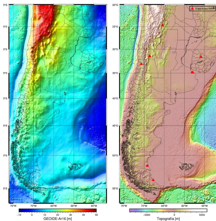
Modelo de geoide argentino GEOIDE- Ar16.
