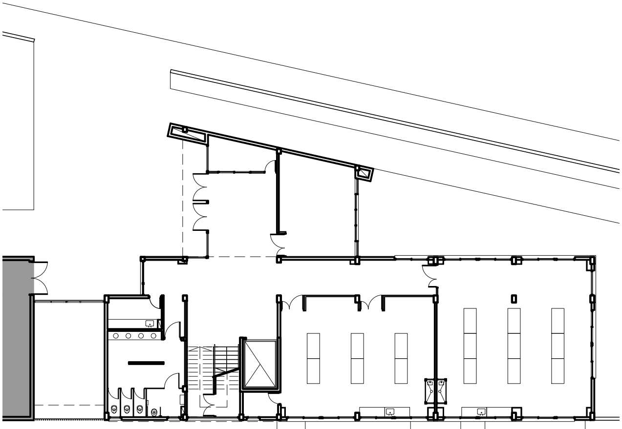
PLANTA BAJA
