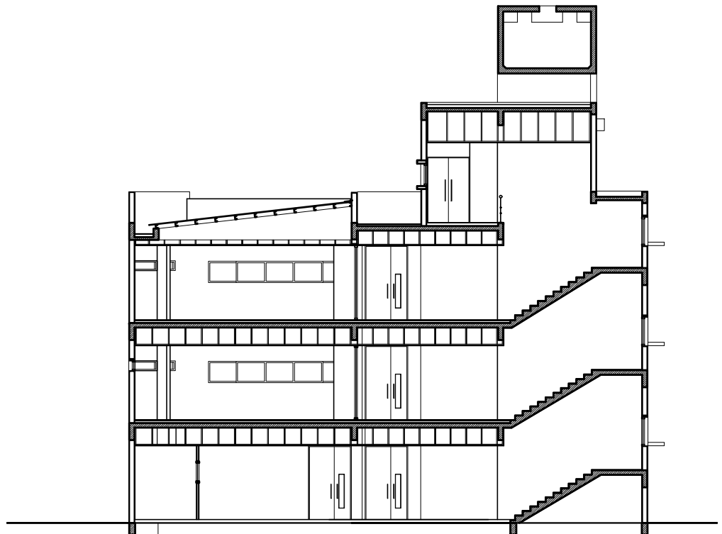
SECCIÓN TRANSVERSAL POR NÚCLEO VERTICAL
