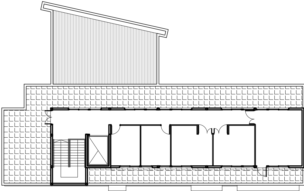
PLANTA TERCERA
