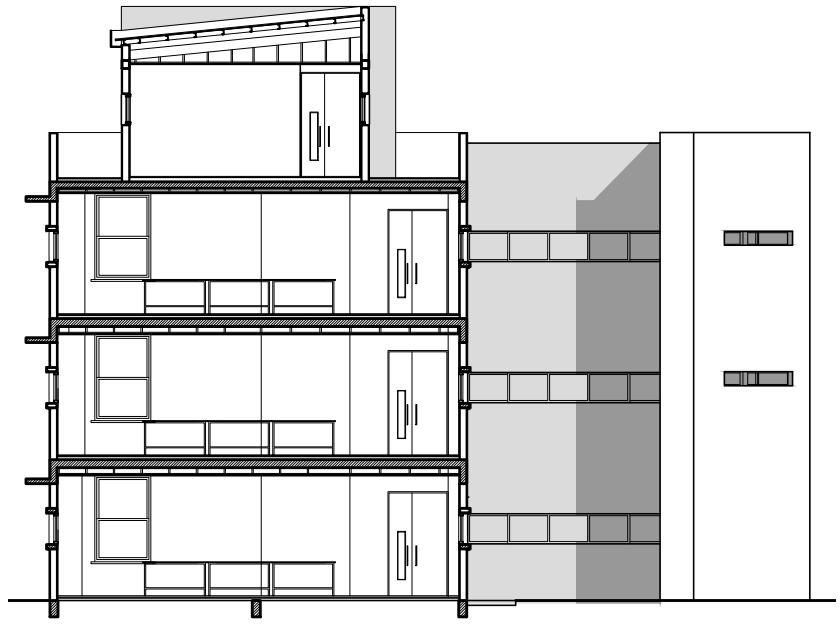
SECCIÓN TRANSVERSAL
