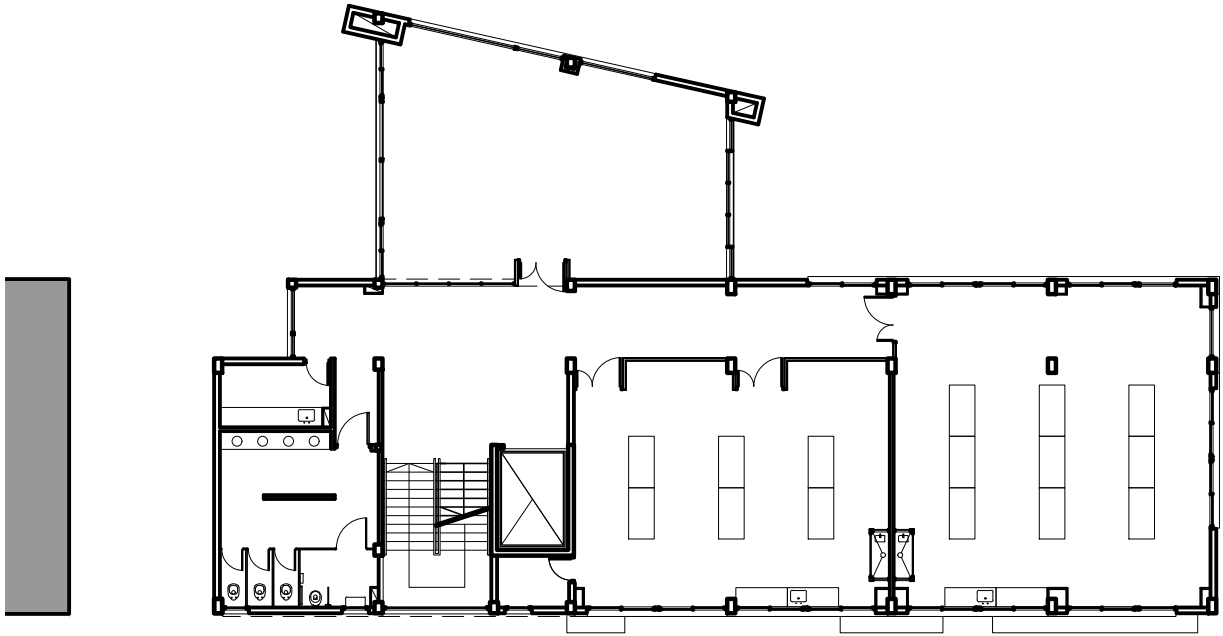
PLANTA SEGUNDA
