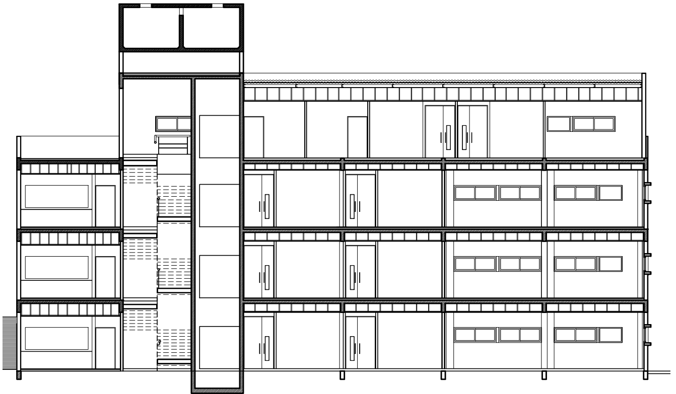
SECCIÓN LONGITUDINAL
