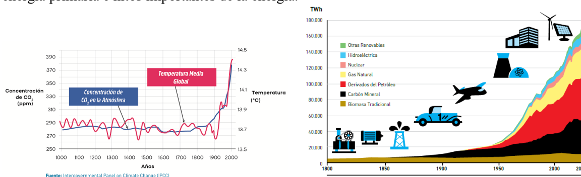
Figura 3a. Concentración de \text{CO}_2 vs. Temperatura media global en función del tiempo. Fuente IPCC.
