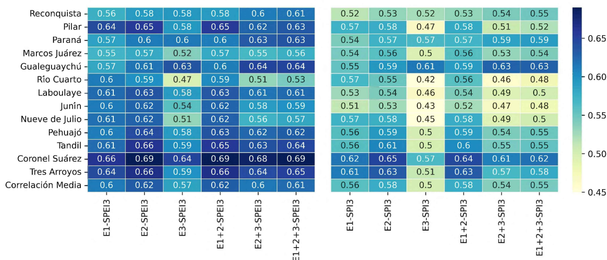
Figura 3: Correlación de Pearson entre las anomalías de humedad del suelo y los índices a) SPEI-3 y b) SPI-3 para las 14 estaciones meteorológicas, ordenadas de norte a sur, en el período 1981-2020. Las siglas E1, E2, E3, E1+2, E2+3 y E1+2+3 representan los espesores 1 (0-7 cm), 2 (7-28 cm) y 3 (28-100 cm), y la combinación de espesores 1 y 2, 2 y 3, y 1,2 y 3 respectivamente.
