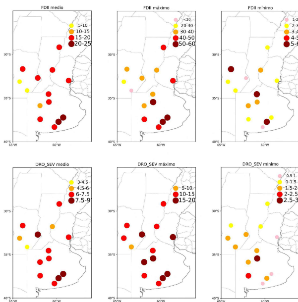
Figura 5: Distribución espacial de los valores de Índice FDII (ec. 3) a) medio, b) máximo y c) mínimo y término DRO_SEV (ec. 2) d) medio, e) máximo y f) mínimo en las 14 estaciones meteorológicas seleccionadas. Los umbrales corresponden a los cuartiles de los valores medios, máximos y mínimos del término DRO_SEV y del índice FDII.
