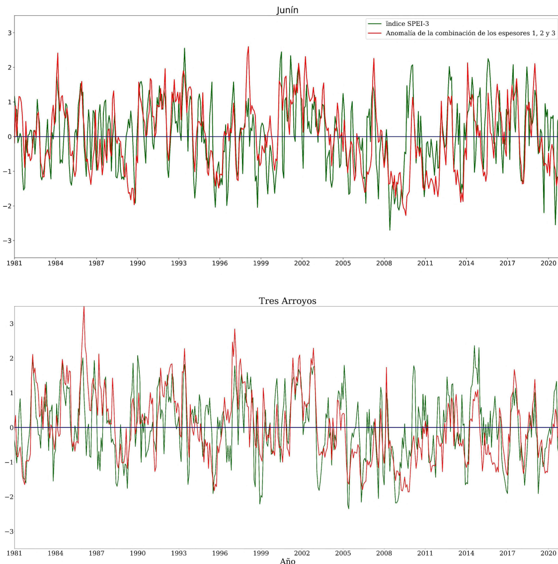
Figura 4: Series temporales de anomalías de humedad del suelo para la suma de espesores 1, 2 y 3 y del SPEI-3 para las estaciones de a) Junín y b) Tres Arroyos.
