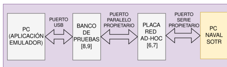
Fig. 1. Esquema de interconexión realizado para el reemplazo de uno de los nodos de un sistema distribuido de tiempo real. SOTR: Sistema Operativo de Tiempo Real.
