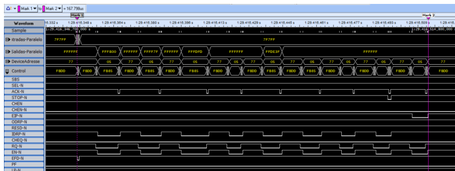
Fig. 10. Captura de analizador lógico de placa de transporte GMD original. Se registra el tiempo entre cursores: 167,798 us.
