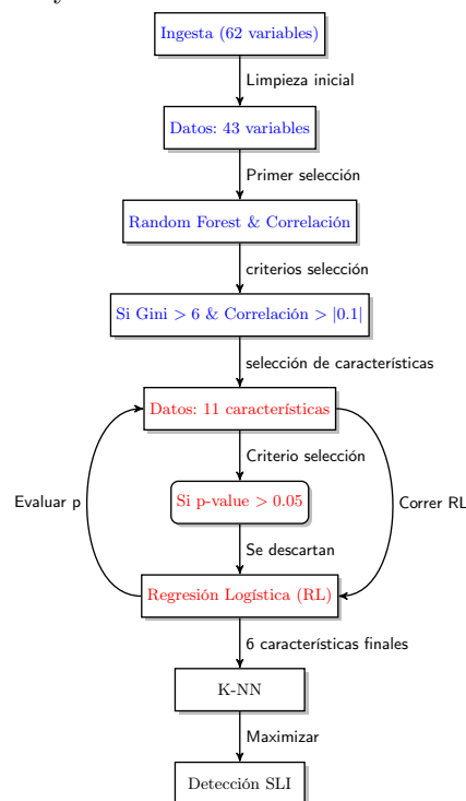
Fig. 1: Pipeline que ilustra la metodología propuesta.
