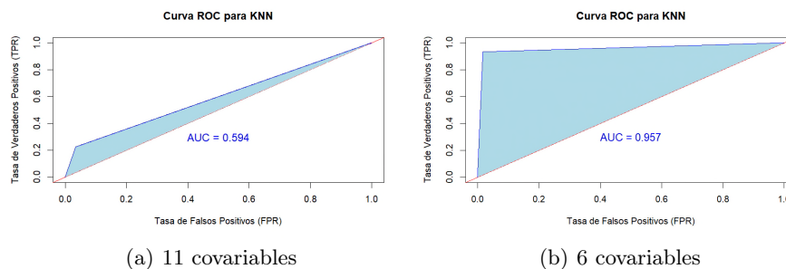
Fig. 4: Resultados del modelo 14-NN para (a) 11 y (b) 6, covariables.
