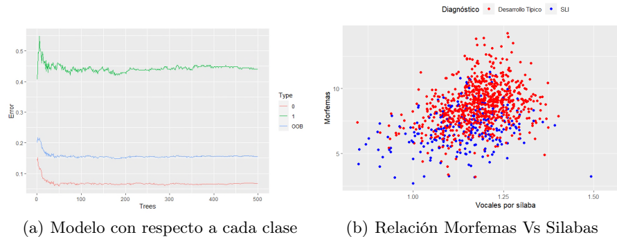
Fig. 2: (a) Comportamiento del modelo con respecto a cada clase de predicción. Observe como los árboles se empiezan a estabilizar a partir del valor 16 aproximadamente, para el tipo 1 (Clase 1) y OOB, mientras que para el tipo 0 (Clase 0), se empieza a estabilizar en 200 aproximadamente. Esta inspección visual permite establecer el valor de los árboles en 500. (b) Relación entre Cantidad de Morfemas por Respuesta y promedio de silabas
