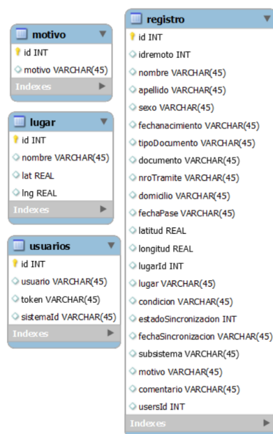
Fig. 9: Diagrama de Entidad de la Base de Datos de la aplicación.
