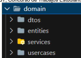
Fig. 7: Directorio “domain” del Proyecto que representa la Capa de Dominio.
