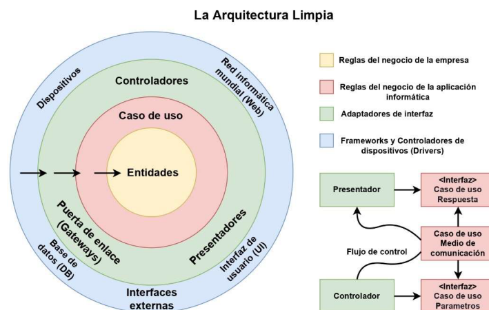
Fig. 2: Gráfico de Arquitectura Limpia según Robert. C. Martin
