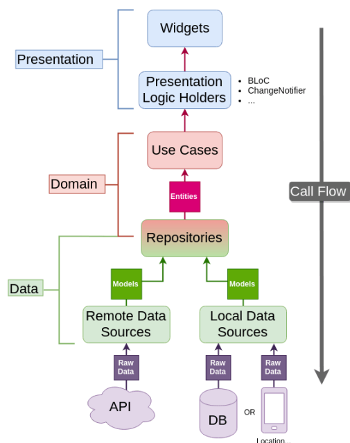
Fig. 3: Modelo del Flujo de llamadas de Clean Architecture adaptado a Flutter por Mahmoud Elbokl
