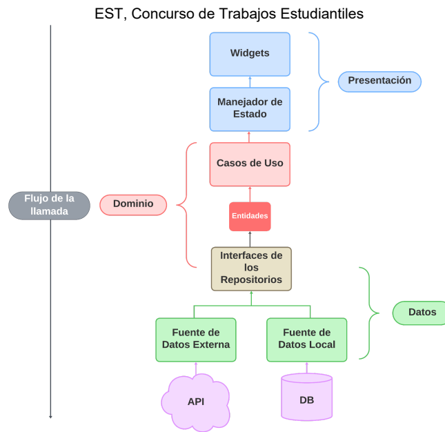
Fig. 4: Modelo adaptado del flujo de llamadas de Clean Architecture para este proyecto.
