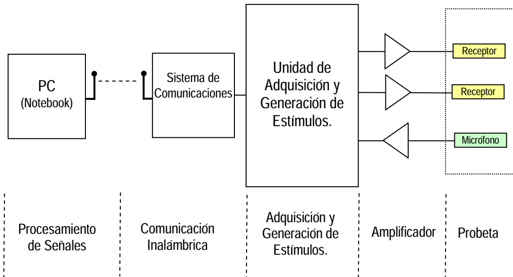
Figura 2. Diagrama en bloques de equipo de OAE.
