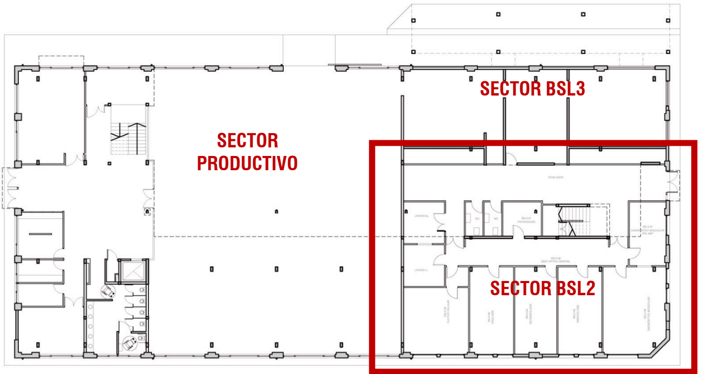
CENTRO DE INVESTIGACIONES BIOLÓGICAS / PLANTA BAJA – SECTOR BSL2
