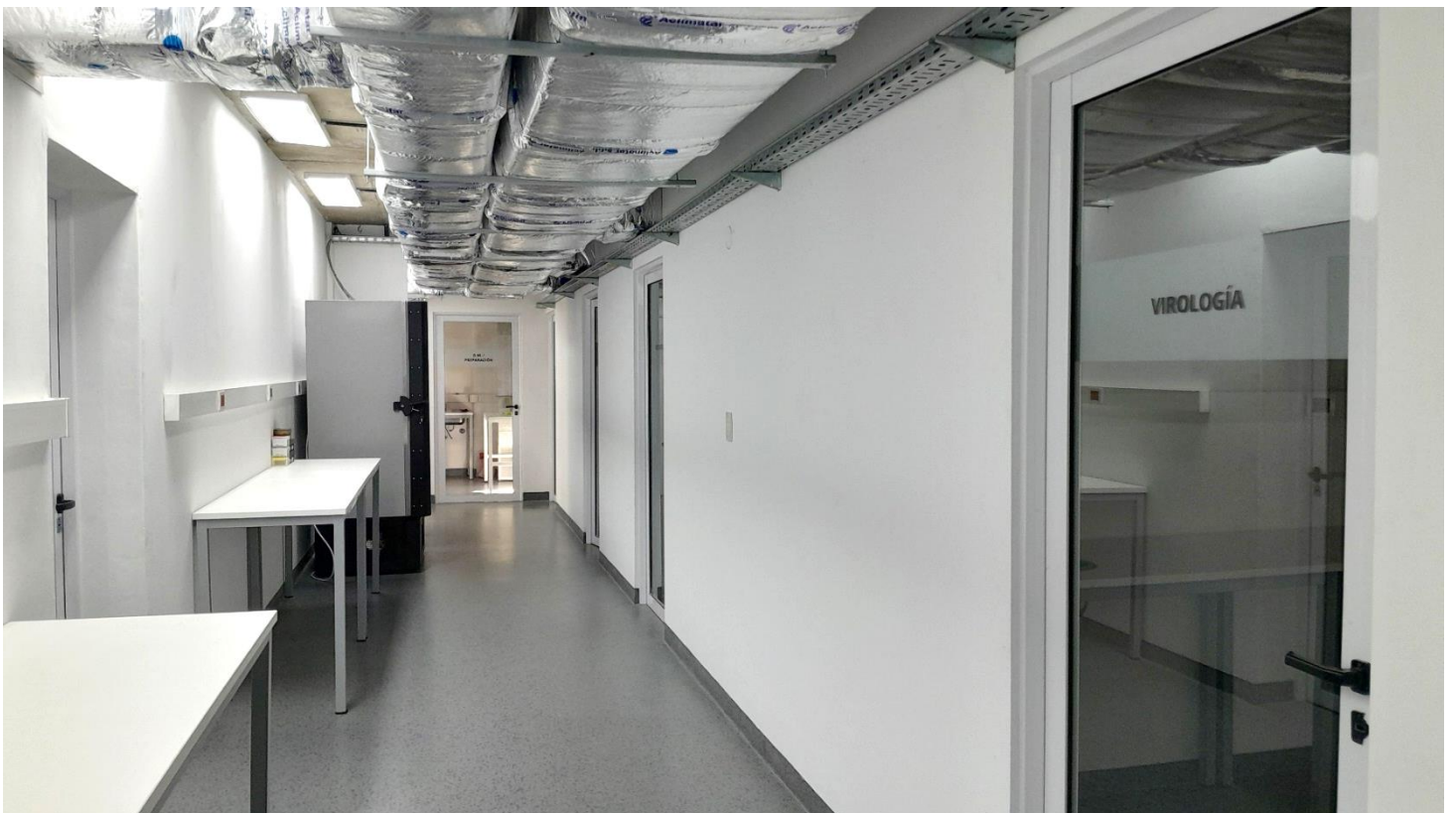
“BACK-OFFICE” / SECTOR COMÚN DE DISTRIBUCIÓN Y SERVICIOS
