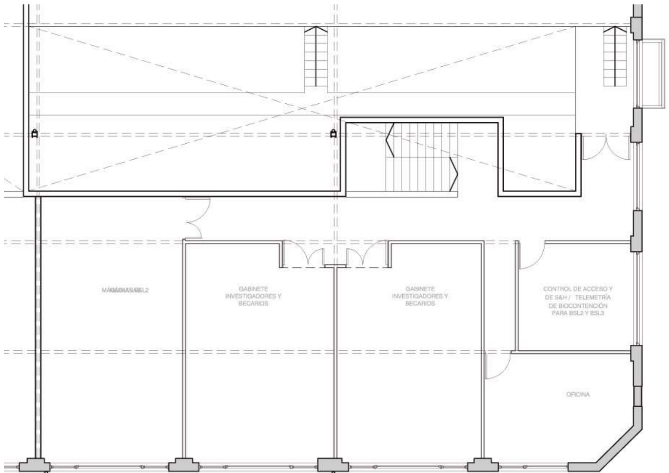
SECTOR BSL2 – PLANTA PRIMERA
