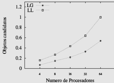
Figura 4.11: Número de objetos candidatos obtenidos al utilizar centros globales versus centros locales sobre la colección de palabras UK.
