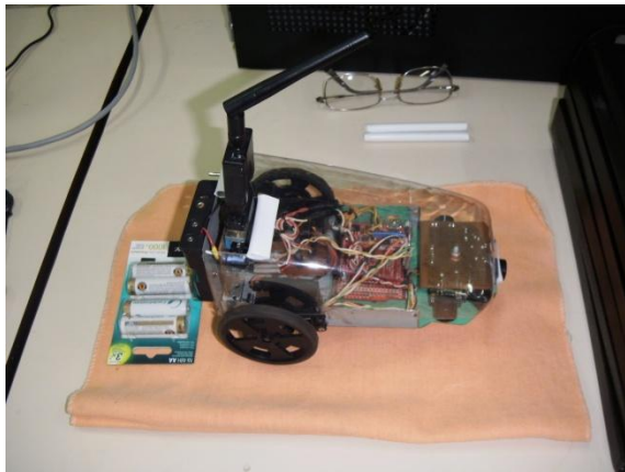
Fig.1 Prototipo con tracción diferencial y un arreglo de cinco sonares y conexión bluetooth
