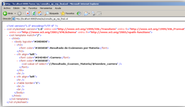
Figura 11: Hoja de estilo cargada al repositorio
