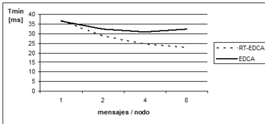
Fig. 5. Período mínimo para 40 mensajes con diferentes agrupamientos
