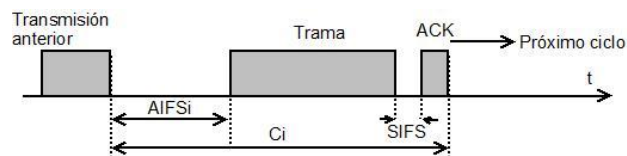
Fig. 2. RT-EDCA: Esquema básico.
