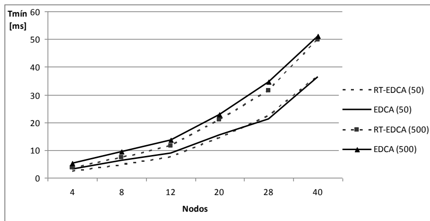
Fig. 4. Período mínimo comparativo entre RT-EDCA vs EDCA
