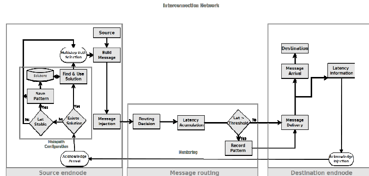
Fig. 3 Algoritmo PR-DRB con todas las fases integradas
