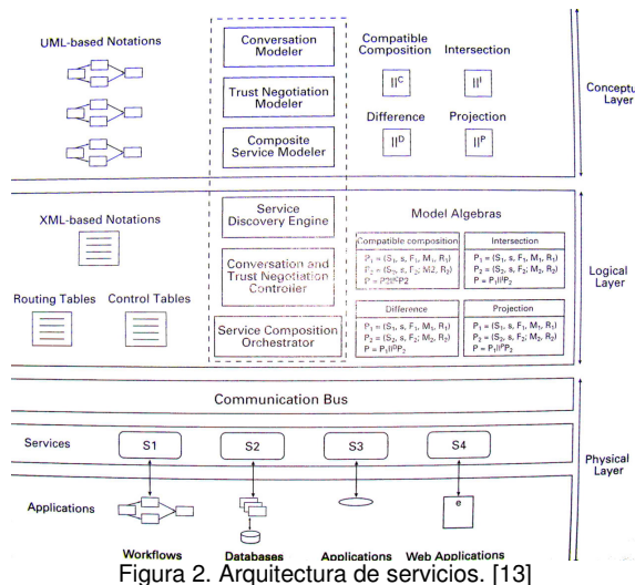
Figura 2. Arquitectura de servicios. [13]
