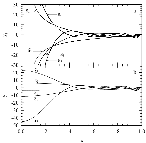
Figura 3.3: a. La autofunción y_1 para los modos g_1, \dots, g_5 con \ell = 1 , correspondientes a un modelo de enana blanca de 0.3 M_{\odot} de helio puro con T_{\text{eff}} = 11900 K. Nótese las grandes amplitudes de tales modos en el núcleo estelar. b. Igual que para el panel a. , pero para el caso \ell = 2 .
