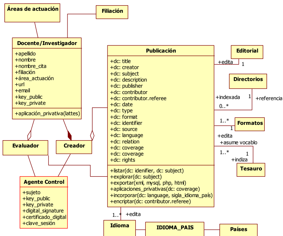
Figura 3 Diagrama de Clases de la Hemeroteca Digital
