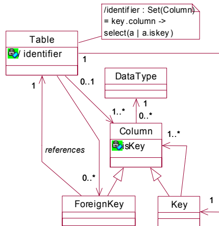
Figura 8. Metamodelo Relacional
