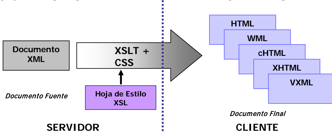
Figura 1- Arquitectura XML
