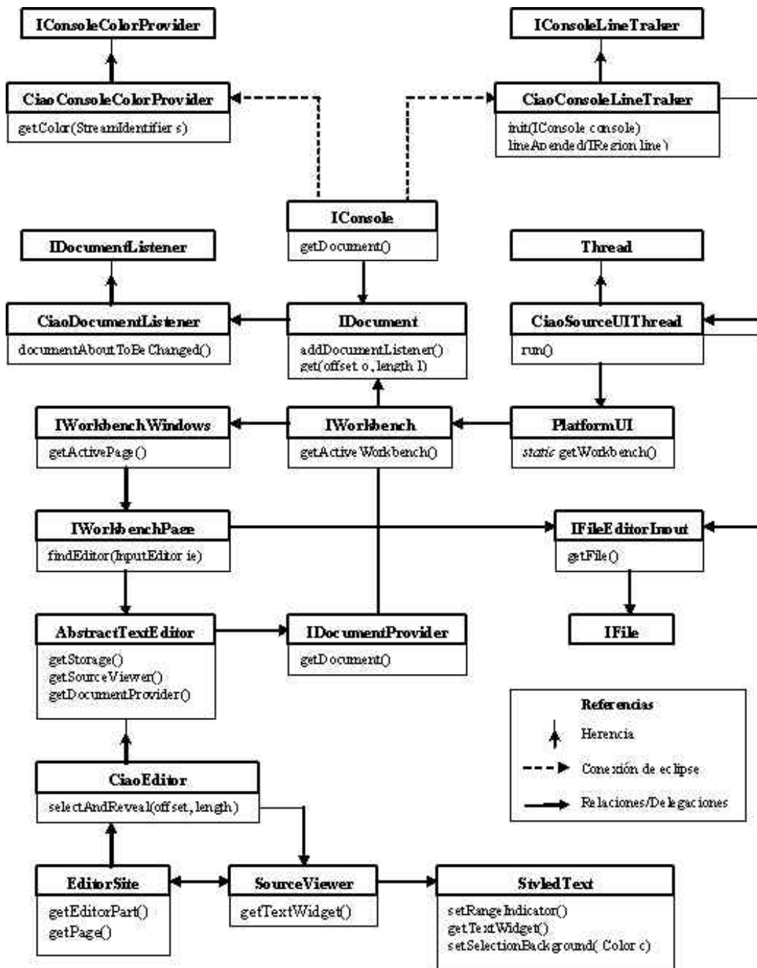
Figura 5: Diagrama de clases relacionadas a la implementación del coloreo de código fuente
