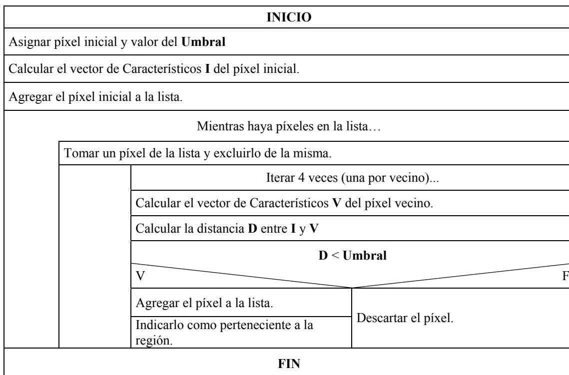
Figura 1: Diagrama de Chapin del algoritmo
