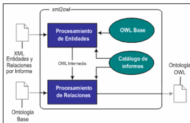
Figura 13 - Arquitectura xml2owl
