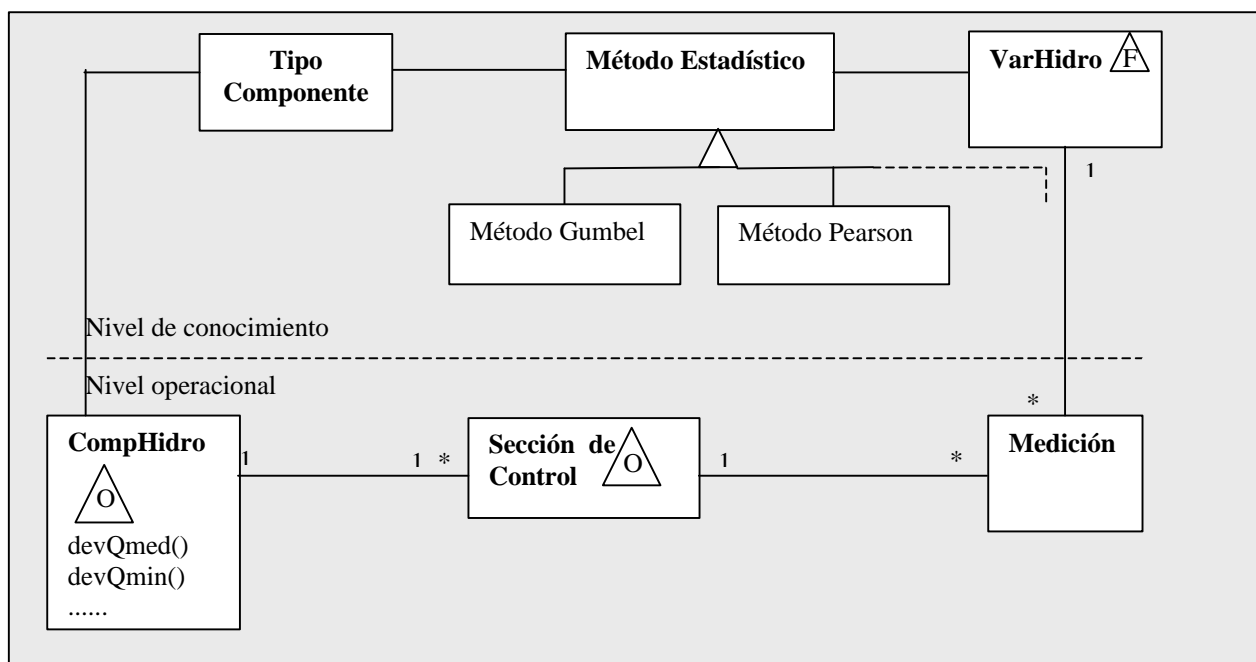
Fig. 11 - Separación de nivel de conocimiento y nivel operacional para tratamiento estadístico
