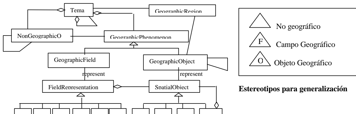
Fig. 3 - Diagrama de clases de GeoFrame
