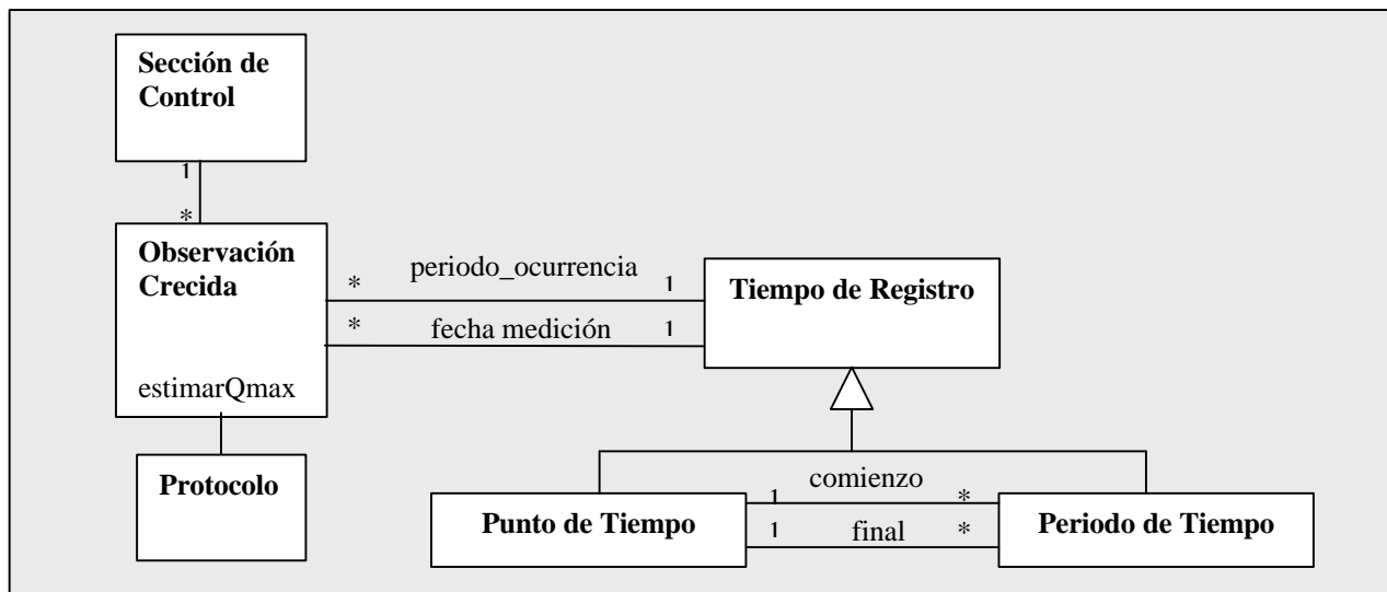
Fig. 10 - Adaptación del Patrón Dual Time Record para registrar eventos observados
