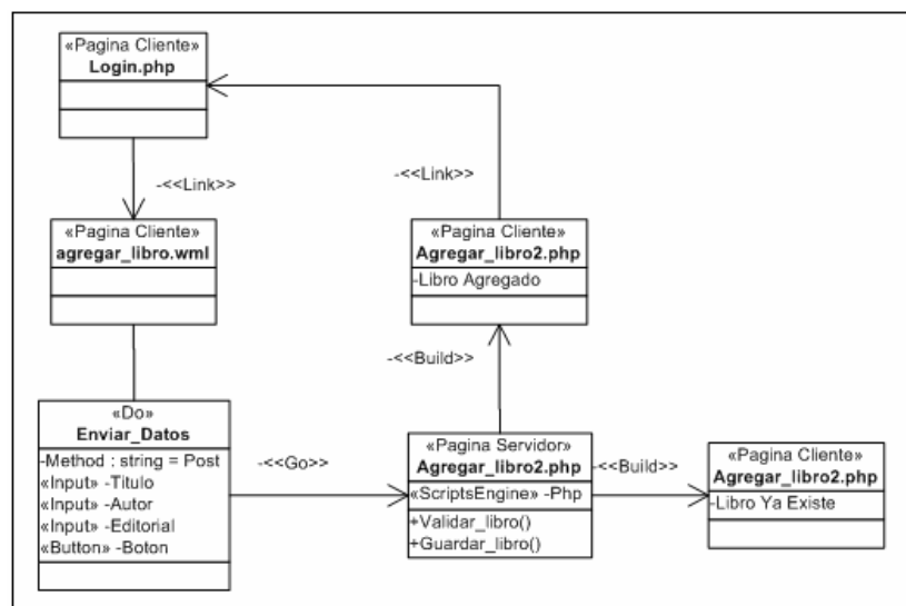
Figura n°8 Diagrama Clases de Diseño: Agregar Libro
