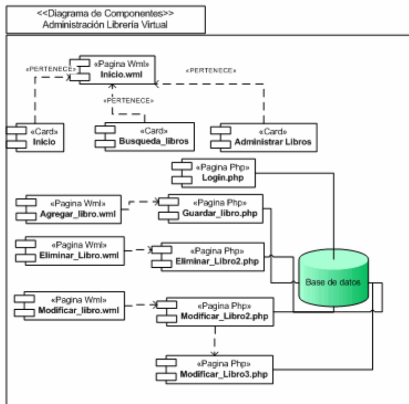
Figura n°7 Diagrama de Componentes Librería Virtual
