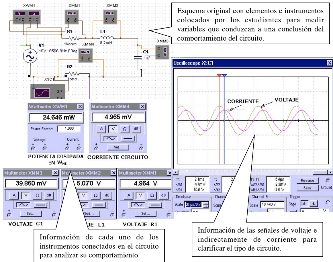
Figura 2. Desarrollo de una práctica de laboratorio por medio de un software de simulación.
