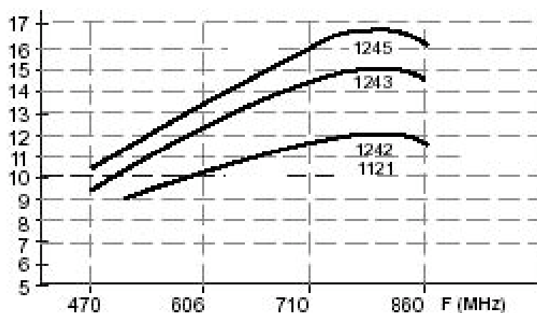
Figura 8: Respuesta en frecuencia de la Antena de UHF Monolítica Ref. 1243.
