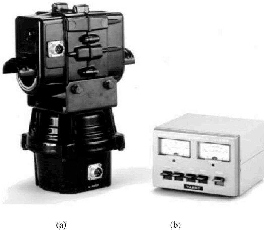
Figura 1: Rotor de antenas G-5500 de Yaesu y controlador
