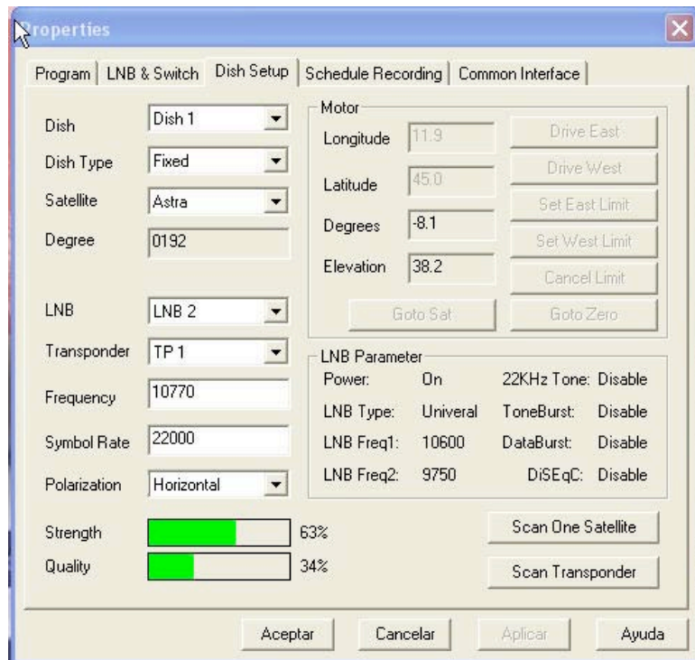
Figura 6: Ventana de propiedades de la Tarjeta PCI de TV satélite con los valores de los parámetros de la señal que recibe la antena parabólica de televisión vía satélite en un canal determinado.
