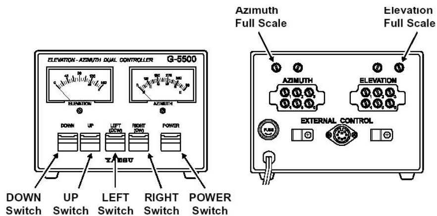
Figura 2: Vista frontal y trasera del controlador del rotor de la Figura 1.
