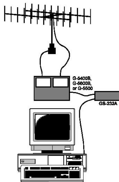
Figura 4: Control remoto del rotor por ordenador mediante la unidad GS-232A.
