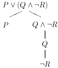
Figura 3: Representación de tableaux mediante lista de ramas.
