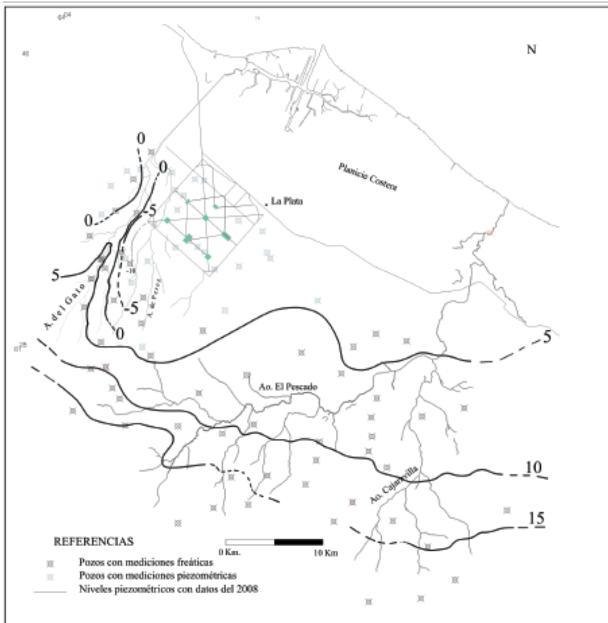
Figura 3: Mapa isofreático. Abril 2008
