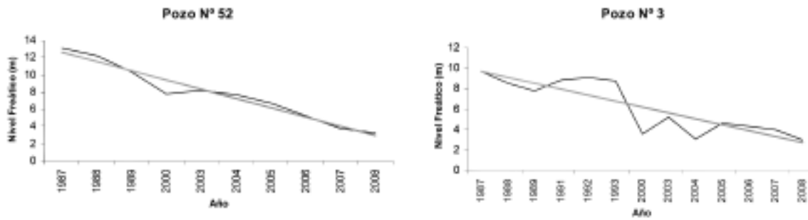
Figura 4: Niveles freáticos, período 1987 - 2008
