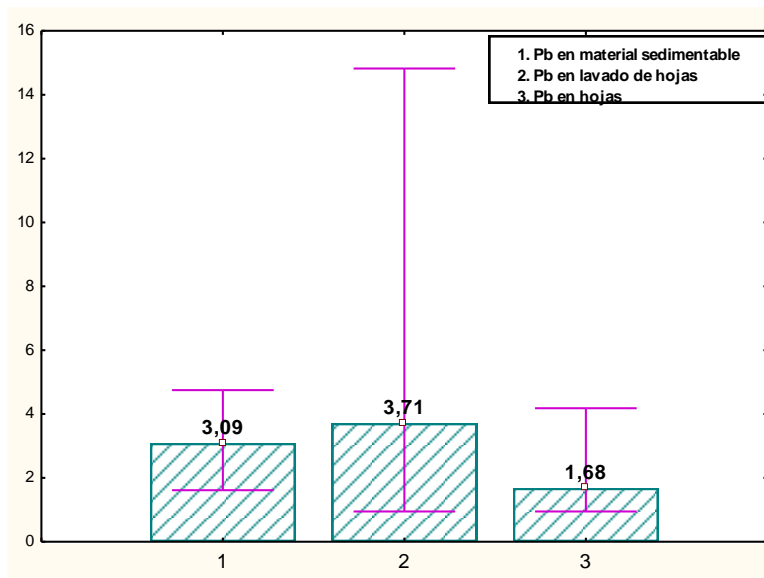
Figura 1. Relaciones de concentración de Pb en los tipos de muestras analizadas respecto a las concentraciones en el sitio de referencia. Se indica valor medio, máximo y mínimo.
