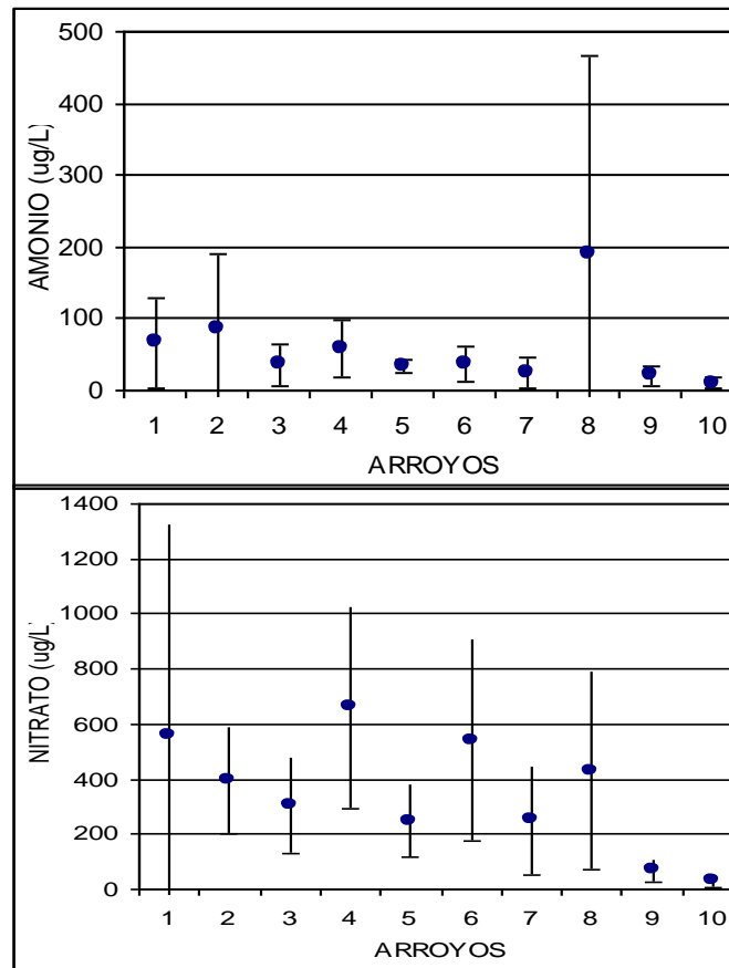
Figura 2. Promedio anual y desvío estándar del amonio y el nitrato en los 10 arroyos. Figure 2. Ammonia and nitrate annual mean and standard deviation at the 10 streams.
