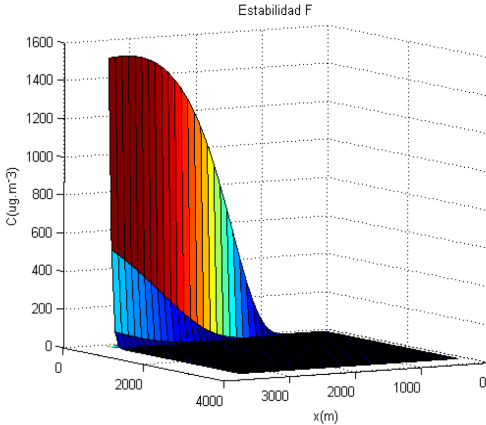
Figura 3. Valores simulados de concentración( \mu\text{g}\cdot\text{m}^{-3} ), estabilidad F, área rural, u=2\text{m}\cdot\text{s}^{-1}
