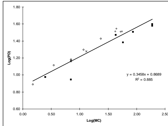
Figura 11.6. Profundidad del dentario debajo del molar carnívoros (PD) en función de la masa corporal en las especies de Carnivora de la Tabla 12.2. Referencias: rombos grises (Hipercarnívoros/H); cuadrados negros (Hipercarnívoros/C); rombos blancos (Mesocarnívoros); cruces (omnívoros).
