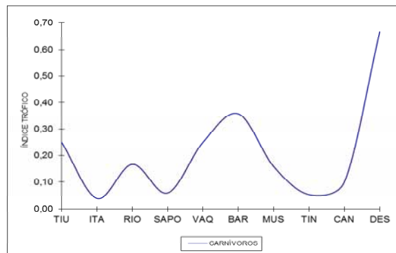
Figura 15.11. Abundancia relativa de carnívoros.
