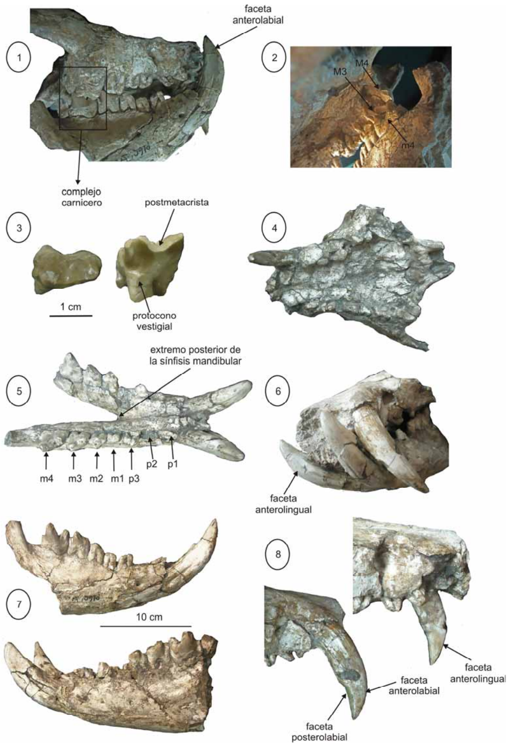
Figura 12.35. Arminiheringia . 1. A. auceta . Vista labial de la porción anterior del cráneo y la mandíbula (MACN 10972 y MACN 10970). 2. Vista lingual del complejo carnicero mostrando la extensión de la faceta de oclusión en los molares superiores de un individuo senil. 3. A. cultrata . Vista oclusal y lingual de un molar superior aislado (MACNA 10974). 4-8. A. auceta . 4. Vista palatal del cráneo. 5. Vista oclusal de la mandíbula. 6. Vista anterolabial de los caninos en oclusión. 7. Vista labial de las hemimandíbulas derecha (arriba) e izquierda (abajo). 8. Vista lingual (arriba) y labial (abajo) de las facetas de oclusión en los caninos superiores.
