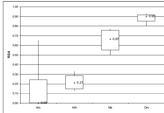
Fig.11.7 Área relativa de molienda. Los rótulos numéricos corresponden a las medianas para cada categoría. H/c, hipercarnívoro (carne); H/h, hipercarnívoro (hueso); Me, mesocarnívoro; Om, omnívoro.
