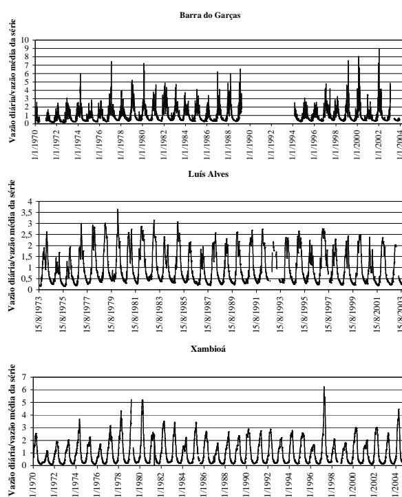
Figura 2. Hidrogramas de vazões diárias normalizados em relação à média da série histórica da estação hidrológica correspondente.
