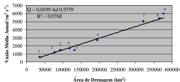
Figura 4. Relação área de drenagem/vazão média anual – compreendendo todas as estações hidrológicas do curso principal do rio Araguaia. 1 – Barra do Garças; 2 – Aruanã; 3 – Bandeirantes; 4 – Luís Alves; 5 – Fazenda Telésforo; 6 – São Félix do Araguaia; 7 – Conceição do Araguaia; 8 – Xambioá; 9 – Araguatins.
