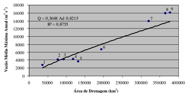
Figura 5. Relação área de drenagem/vazão máxima anual – compreendendo todas as estações hidrológicas do curso principal do rio Araguaia. 1 – Barra do Garças; 2 – Aruanã; 3 – Bandeirantes; 4 – Luís Alves; 5 – Fazenda Telésforo; 6 – São Félix do Araguaia; 7 – Conceição do Araguaia; 8 – Xambioá; 9 – Araguatins.
