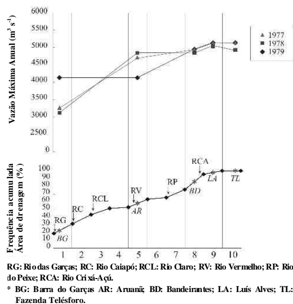
Figura 7. Frequência Acumulada da área de drenagem associada ao tipo de enchente B, ao longo dos dez segmentos do canal do rio Araguaia. ↓ - confluência com os principais afluentes. * - Localização das estações hidrológicas.
