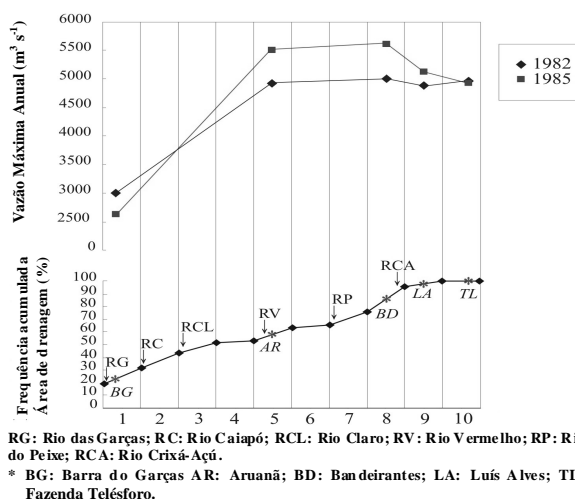
Figura 8. Frequência acumulada da área de drenagem associada ao tipo de enchente C, ao longo dos dez segmentos do canal do rio Araguaia. ↓ - confluência com os principais afluentes. * - Localização das estações hidrológicas.
