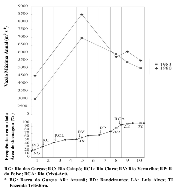
Figura 6. Frequência acumulada da área de drenagem associada ao tipo de enchente A, ao longo dos dez segmentos do canal do rio Araguaia. ↓ – confluência com os principais afluentes. * – Localização das estações hidrológicas.
