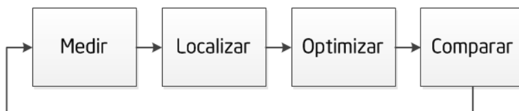
Figura 2.1: Optimización Iterativa
