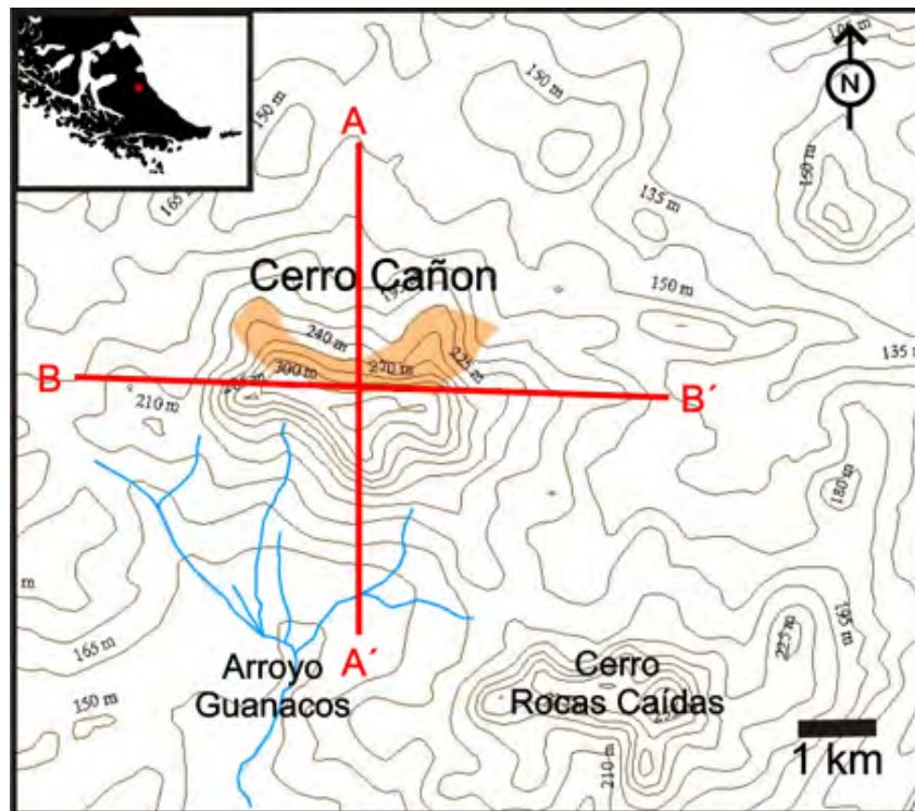
Figura 7.1.7: cerro Cañon. Topografía y ubicación en relación a otros ambientes estudiados en este trabajo. Referencia: líneas rojas: ubicación de los perfiles; área naranja: sector prospectado.
