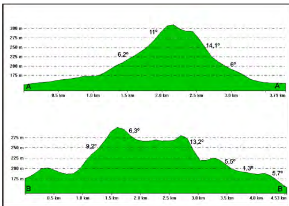
Figura 7.1.8: perfiles en distintos sectores del cerro Cañon.
