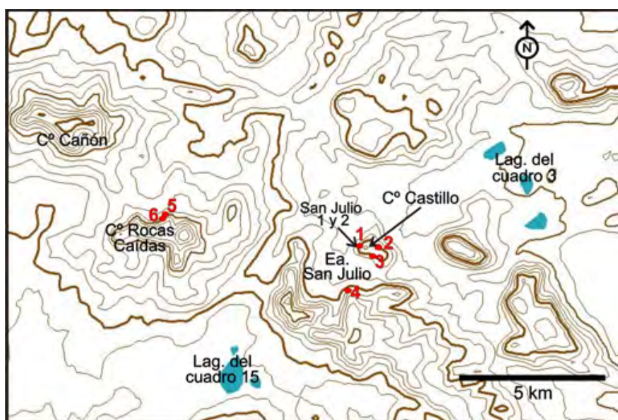
Figura 7.1.59: ubicación de aleros formados en los afloramientos del Terciario en las localidades San Julio y Rocas Caídas.
