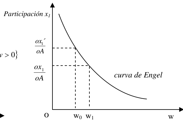
Gráfico 2: Curva de Engel
