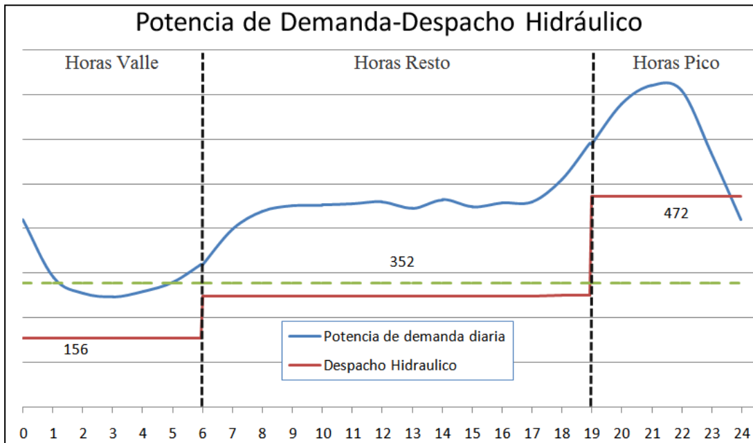
Fig. 3: Potencia de demanda y despacho hidráulico.
