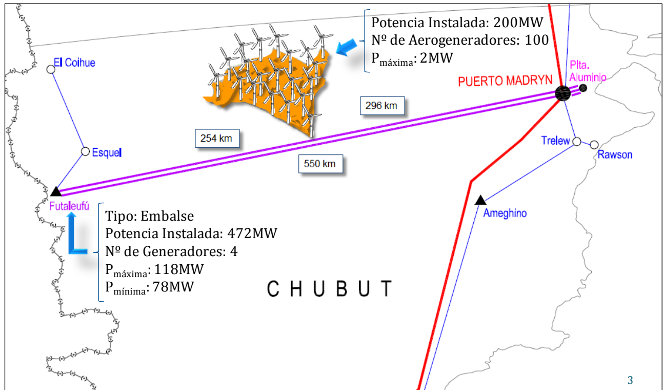
Fig. 1: Unifilar geográfico del área en estudio
