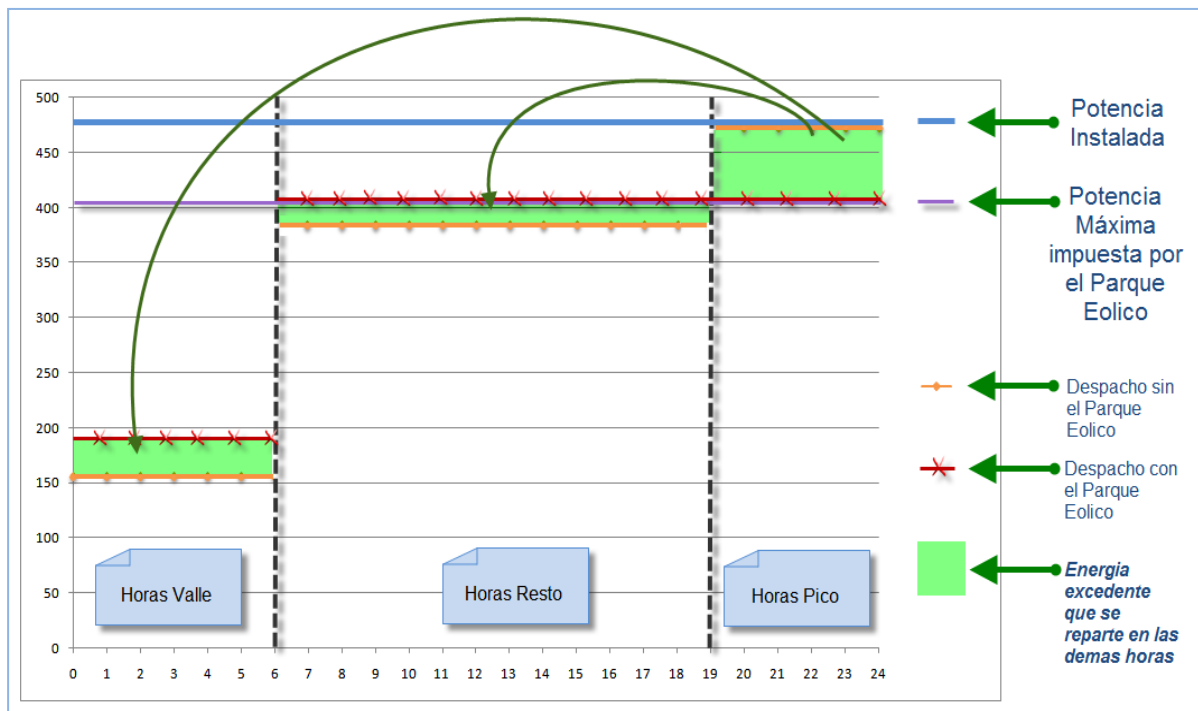
Fig. 4: Despacho hidráulico con y sin generación eólica.
