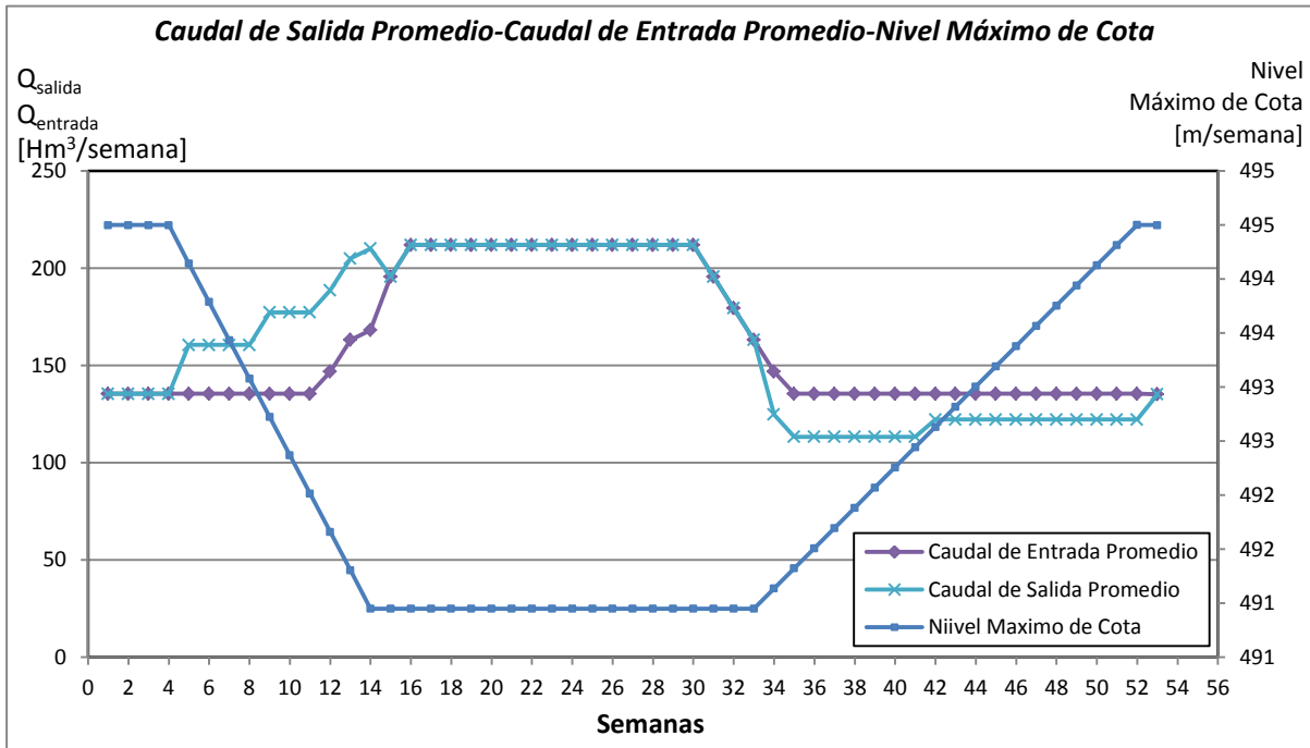
Fig. 2: Caudales de entrada y salida y cota del embalse.
