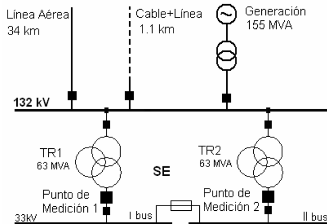
Fig.1: Esquema general de la S.E. y ubicación de los puntos de medición
