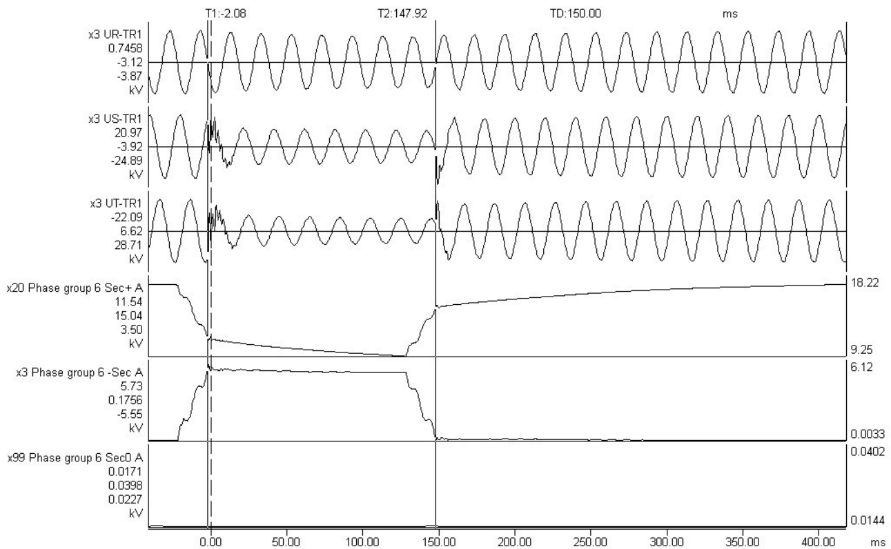
Fig.3. Componentes de secuencia de la tensión. Falla 18/09/2007
