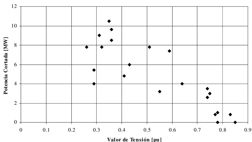
Fig. 5: Potencia cortada en función del valor de la tensión en el complejo.
