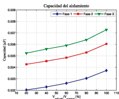
Fig. 1 – Curva de capacidad
