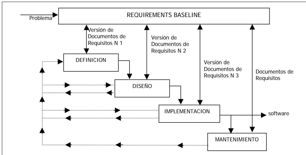
Fig. 2.1 Relación entre Requirements Baseline y el proceso de desarrollo de software [Leite'95]
