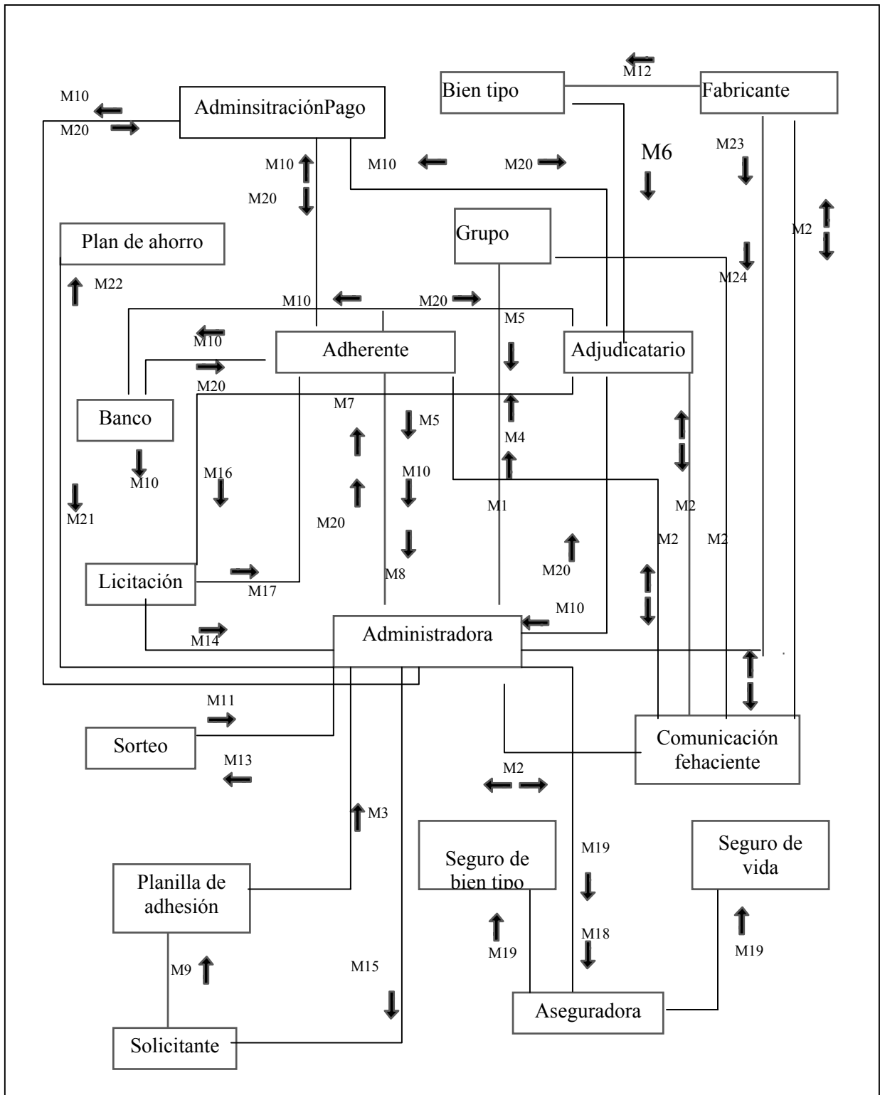
Fig. 8.4: Diagrama de Interconexión
