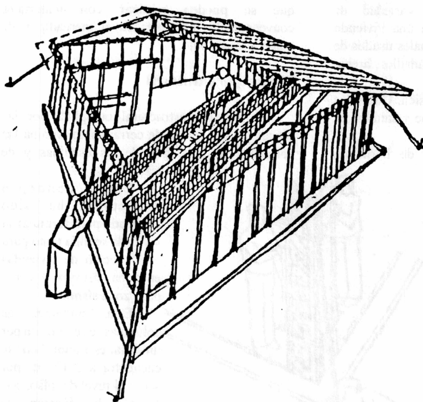
Figura 7: Colocación de techo.
