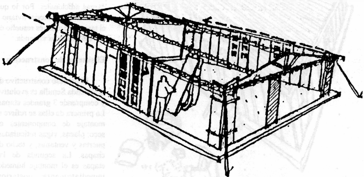
Figura 5: Cerramiento perimetral de placas y ventanas.
