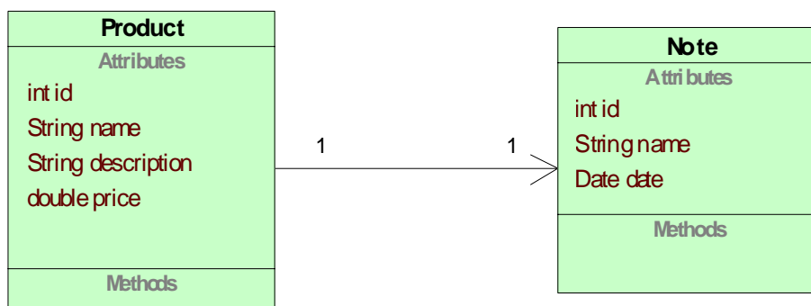
Figura 14 – Relación de 1 a 1(Unidireccional)
