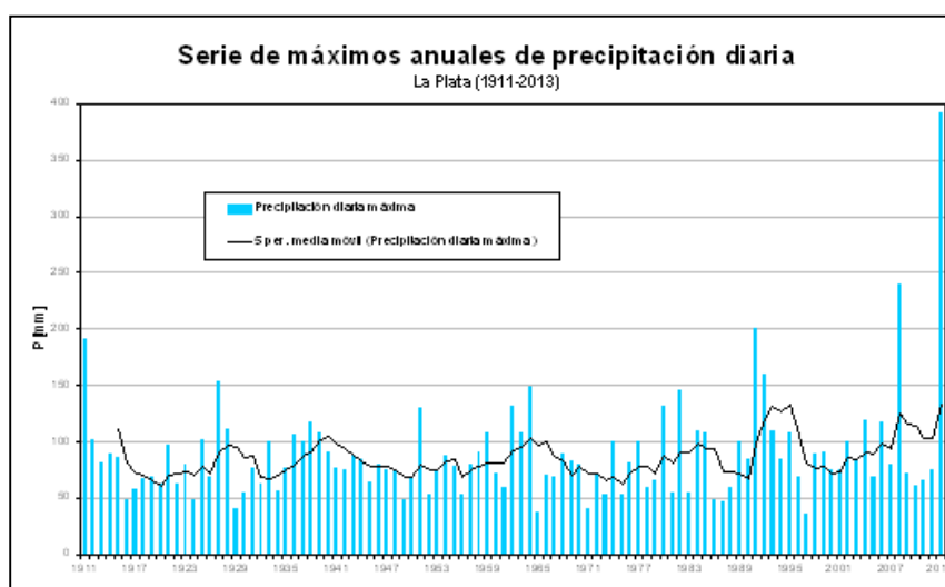
Figura 4 – Serie de precipitaciones diarias máximas [mm] en el período 1911-2013
