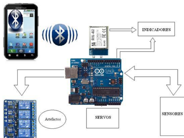
Fig.4 Diagrama de funcionamiento general.
