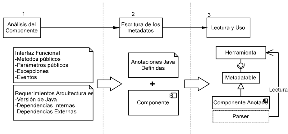
Fig. 2. Aplicación del sistema de metadatos para composición dinámica.
