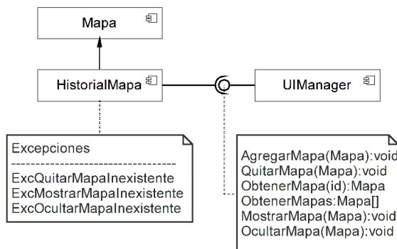
Fig. 3. Parte del diagrama de componentes de la LPS que involucra al componente HistorialMapa
