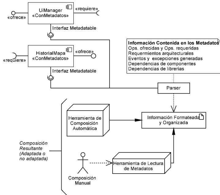
Fig. 4. Proceso de lectura y utilización de los metadatos para composición manual y automática.
